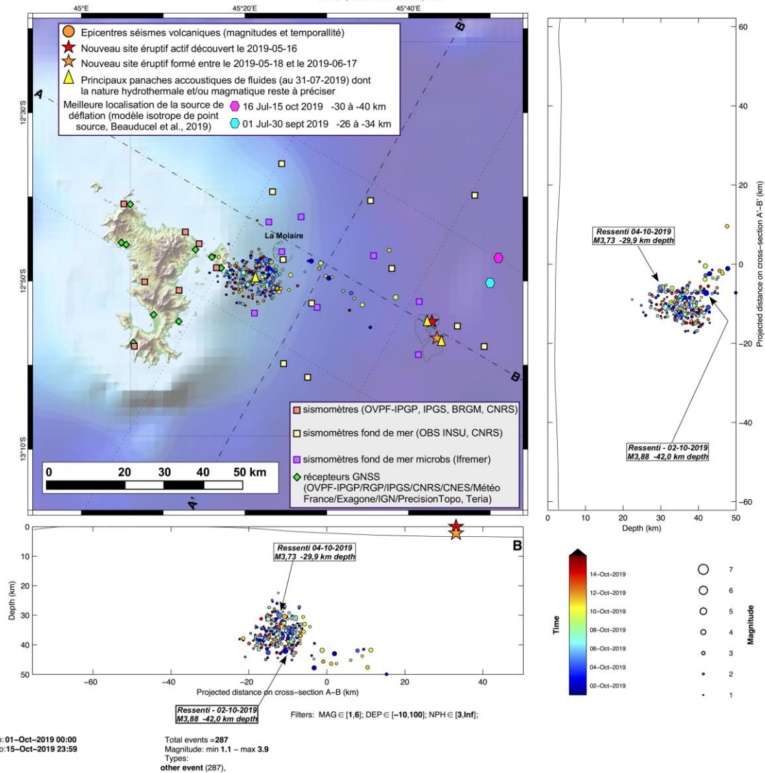
Figure 3: Carte de localisation des épicentres ( \pm 5 km) des séismes volcano-tectoniques avec les réseaux sismiques à terre (IPGP-IFREMER-CNRS-BRGM-BCSF-RéNaSS, IPGS) entre le 1 et le 15 octobre 2019 (15 jours) (échelle temporelle de couleur) et coupes transversales et axiales le long de la ride montrant la localisation estimée en profondeur (précision variant entre \pm 5 km et \pm 15 km) des séismes en fonction de la magnitude (taille des symboles). La localisation approximative des panaches acoustiques identifiés pendant les campagnes océanographiques IFREMER (MD220-Mayobs-1, MD221-Mayobs-2, MD222-Mayobs-3, MD223-Mayobs-4) et dont la nature hydrothermale et/ou magmatique reste à préciser, est indiquée par des triangles jaunes, l'étoile rouge indique le site éruptif nouvellement identifié le 16 mai 2019, et l'étoile orange le deuxième site éruptif identifié le 17 juin 2019. Les structures volcaniques de la zone dite de « La Moltaire » sont indiquées en grisé tout comme les coulées de lave du site éruptif actuel. La position des meilleurs modèles de source en déflation (dégonflement) issues des modélisations (modèle isotrope point source) sur des périodes de temps choisies est indiquée par des polygones de couleur (rose : 2019-07-16/2019-10-15 ; bleu : 2019-07-01/2019-09-30) avec la profondeur associée en km. Les stations sismiques du réseau terrestre, les sismomètres fond de mer (OBS) et les stations de positionnement par satellite GPS sont indiquées par des symboles (voir légende) (© OVPF-IPGP, BRGM, IFREMER, CNRS, BCSF-RéNaSS, IPGS / REVOSIMA).
