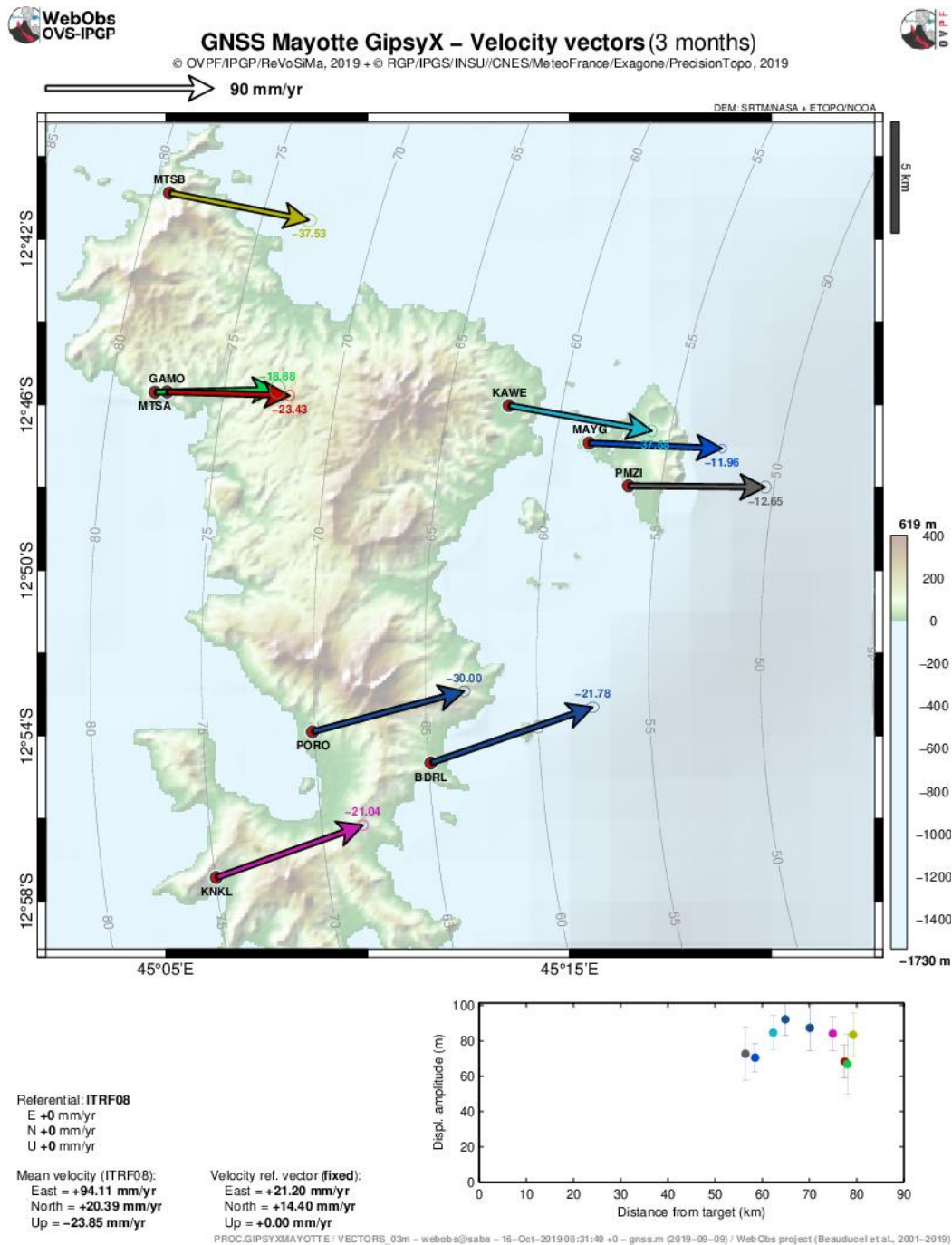
Figure 4 : Déplacements du sol enregistrés sur les stations GPS de Mayotte au cours des 3 derniers mois du 16-07-2019 au 15-10-2019. Les déplacements horizontaux sont représentés sous forme vectorielle et les déplacements verticaux sont indiqués par les valeurs chiffrées en couleur. Post-traitement de ces données réalisé par l'IPGP (@OVPF-IPGP / REVOSIMA).
