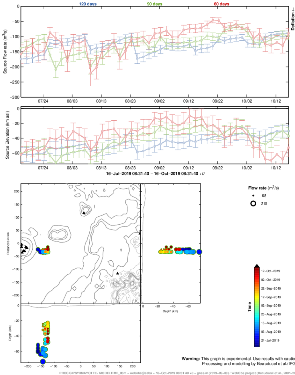
Figure 7 : Évolution spatio-temporelle du meilleur modèle de la source des déformations sur les trois derniers mois. Attention ce graphique ne prend pas en considération les incertitudes du modèle. Chaque point du graphe correspond au résultat d'une modélisation de la source prédominante calculée à partir des données GPS sur une période intégrée de 60 jours (rouge), 90 jours (vert) ou 120 jours (bleu). Le graphe supérieur indique le débit magmatique estimé (en mètres cube par seconde). Le graphe intermédiaire indique la profondeur de la source (en km sous le niveau de la mer). Le graphe inférieur représente les projections horizontale (vue du dessus) et verticales (vues du sud et de l'est) des sources, la taille de chaque marqueur correspondant au débit magmatique ("Flow rate"), et la couleur à la date la plus récente des données utilisées pour chaque modèle (bleu foncé = 16 juillet 2019, rouge foncé = 15 octobre 2019). Les barres d'erreur indiquent l'écart de l'incertitude sur les paramètres à 68% de probabilité. Modélisations réalisées par F. Beauducel (IPGP/IRD) et OVPF-IPGP (©REVOSIMA).
