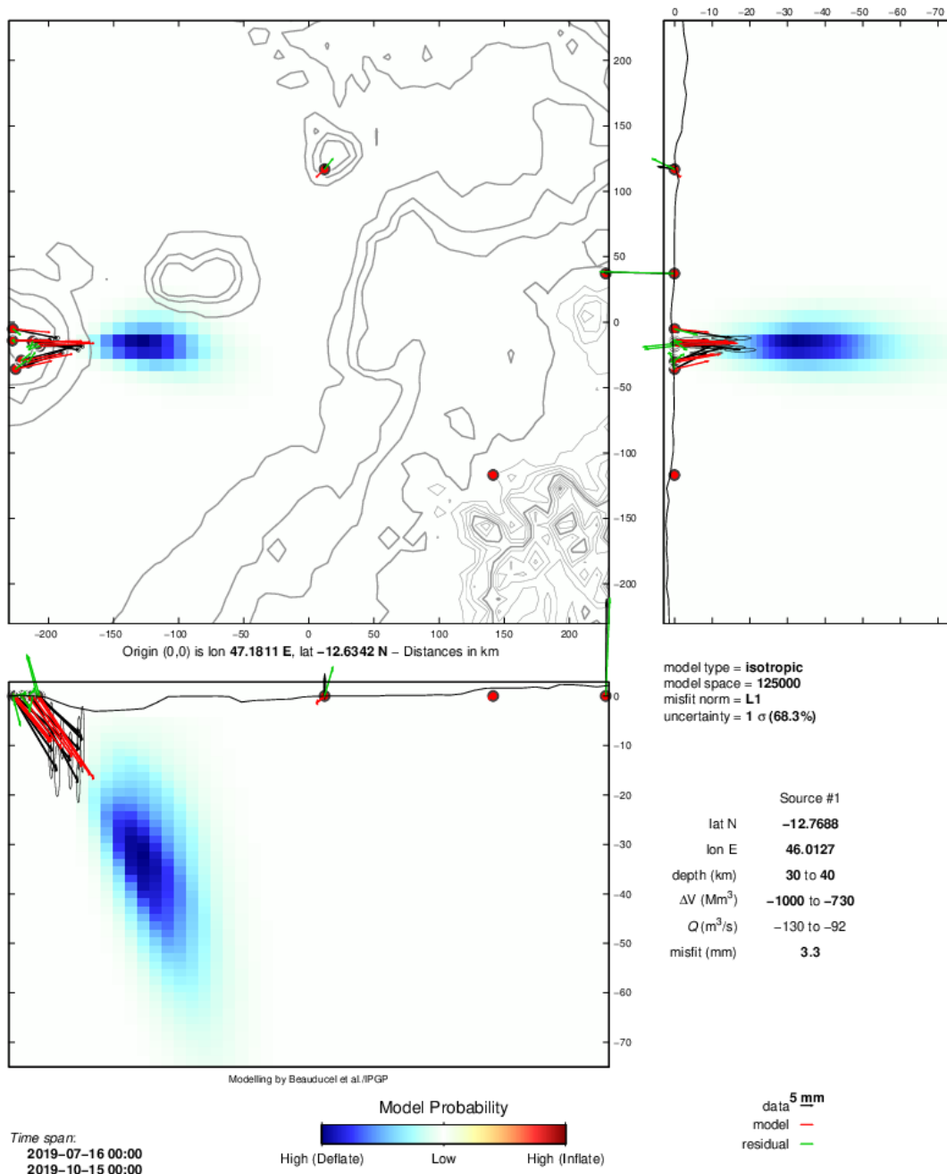
Figure 6: Localisation de la source modélisée (meilleur modèle issu d’une modélisation de type isotrope point source) potentiellement à l’origine des déplacements enregistrés, au cours de la période : 16 juillet - 15 octobre 2019, sur les stations GPS de Mayotte, Grande Glorieuse et DSUA (Madagascar). Les vecteurs en noirs représentent les données observées, les vecteurs en rouge représentent les données modélisées, et les vecteurs en vert représentent les résidus du signal qui n’ont pas pu être modélisés. L’échelle de couleur donne la probabilité en % de la localisation d’une source en déflation (dégradé de couleurs froides, bleus) ou en inflation (dégradé de couleurs chaudes, jaune-rouge) en latitude-longitude et en profondeur selon une représentation cartographique et en coupes verticales orientées est-ouest et nord-sud. Le modèle permet d’estimer la variation de volume de la source, en millions de m 3 (Mm 3 ) et son incertitude, qui explique au mieux les signaux enregistrés. En faisant l’hypothèse que cette variation de volume traduit des transferts de magma dans la lithosphère, le modèle permet d’avoir une estimation préliminaire du flux en m 3 /s de magma associé à la déflation. Modélisations réalisées par F. Beauducel (IPGP/IRD) et OVSP-IPGP (©REVOSIMA).
